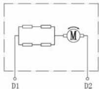
接线图
